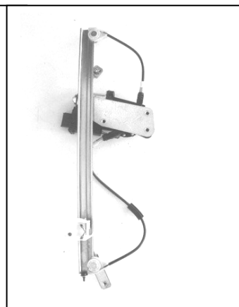
Nostro alzacristallo – our window regulator – notre lève-vitre – unser Fensterheber – nuestro elevalunas – nosso levantador de vidro – bizim cam acacagi - Γρύλος δικός μας
