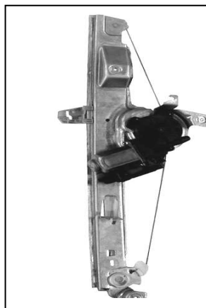
Alzacristallo originale – oem window regulator – lève-vitre original – Fensterheber von oem – elevalunas original – levantador de vidro original – orijinal cam acacagi - Γρύλος γνήσιος
