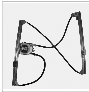
Alzacristallo originale – oem window regulator – lève-vitre original – Fensterheber von oem – elevallas original – levandator de vidro original orijinal cam acacagi - Γρύλος γνήσιος
