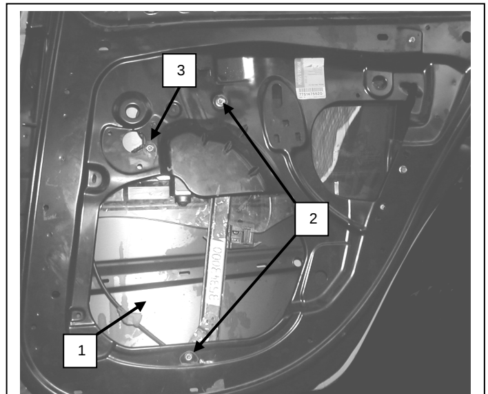
Porta lato destro, Portière avant droite, Right front door, Puerta lado derecho, Vorne rechte Tür, Porta frente dirieta, Sag on kapi, πόρτα εμπρός δεξιά
