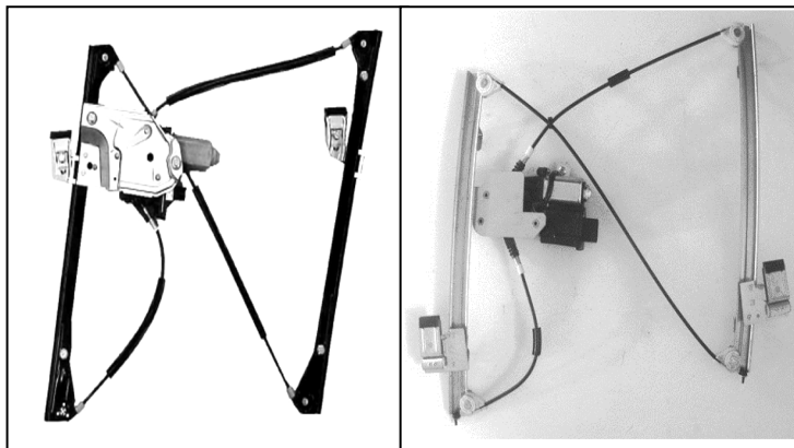
Alzacristallo originale – oem window regulator – lève-vitre original – Fensterheber von oem – elevallunas original – levandator de vidro original – orijinal cam acacagi - Γρύλος γνήσιος
