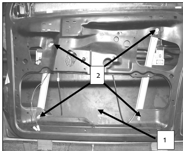
Porta lato destro, Portière avant droite, Right front door, Puerta lado derecho, Vorne rechte Tür, Porta frente dirieta, Sag on kapı, πόρτα εμπρός δεξιά
