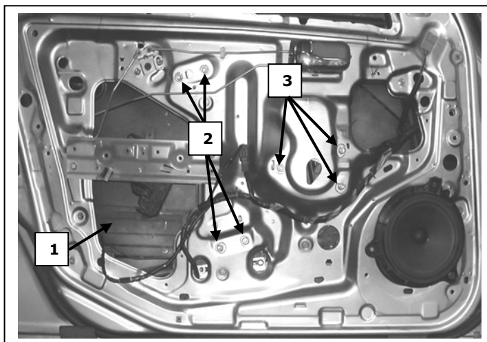
Porta lato destro, Portière avant droite, Right front door, Puerta lado derecho, Vorne rechte Tür, Porta frente dirieta, Sag on kapı, νότια εμπρόσθια δεξιά
