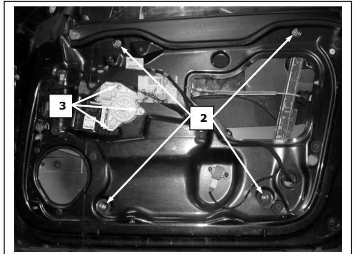
Porta lato destro, Portière avant droite, Right front door, Puerta lado derecho, Vorne rechte Tür, Porta frente dirota, Sag on kapi, πόρτα εμπρός δεξιά
