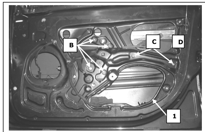
Porta lato destro, Portière avant droite, Right front door, Puerta lado derecho, Vorne rechte Tür, Porta frente dirieta, Sag on kapi, πόρτα εμπρόςθια δεξί
