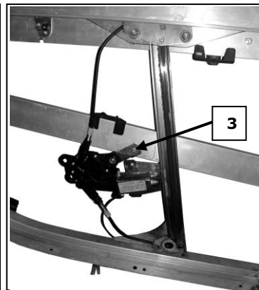
Porta lato sinistro, Portière avant gauche, Left front door, Puerta lado izquierdo, Vorne links Tür, Porta frente esquerda, Sol on kapi, πόρτα εμπρός/αριστερή
