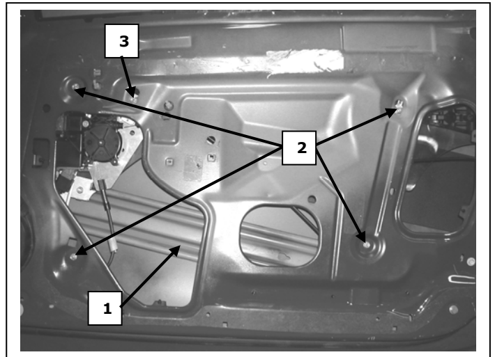
Porta lato destro, Portière avant droite, Right front door, Puerta lado derecho, Vorne rechte Tür, Porta frente dirieta, Sag on kapi, νόρτα εμπρόςθια δεξιά
