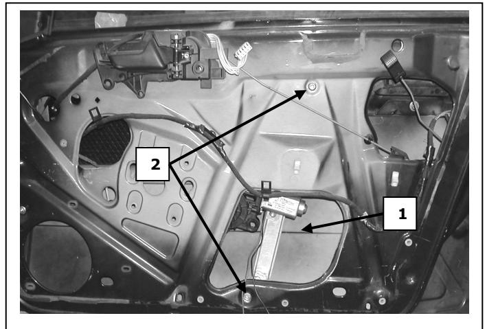
Porta lato destro, Portière avant droite, Right front door, Puerta lado derecho, Vorne rechte Tür, Porta frente direita, Sag on kapi,
