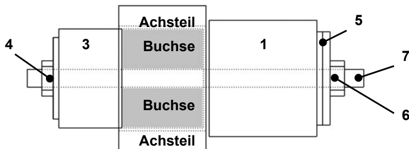
Werkzeug vorgespannt; Beginn der Buchsen-Demontage
