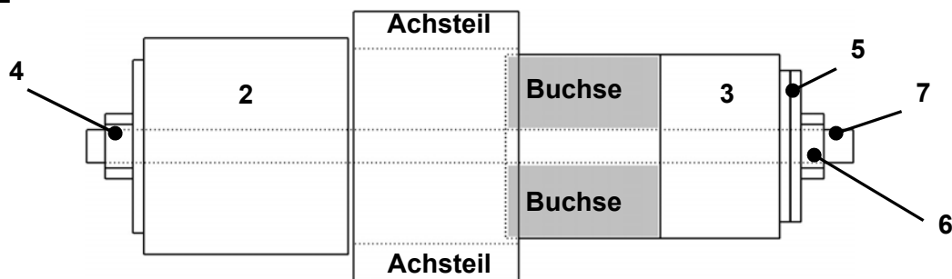
Werkzeug vorgespannt; Beginn der Buchsen-Montage
