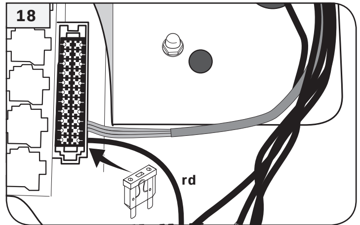
Sicherungskasten fusebox
